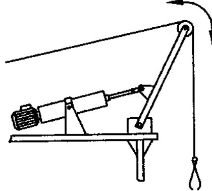
Commande d'inclinaison de bras de manutention
