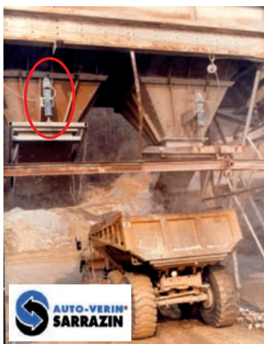
Auto-vérin de commande de casque de trémie
